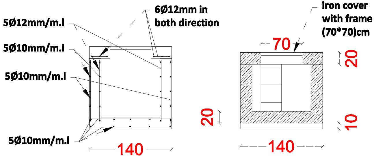
Manhole (140*140)cm
