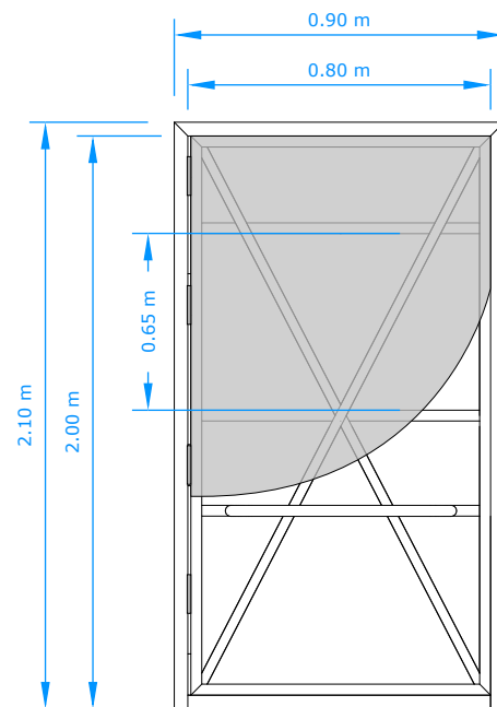
02 B WC / STORAGE DOOR SCALE 1:30
