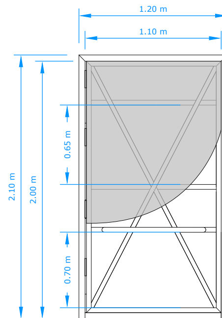
01 B PWSN WC DOOR SCALE 1:30
