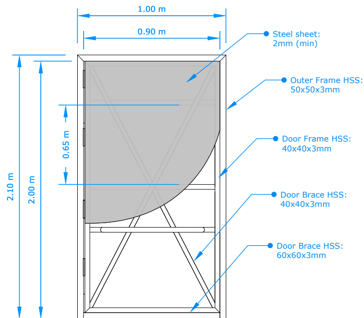
03 B0 STANDARD DOOR SCALE 1:30
