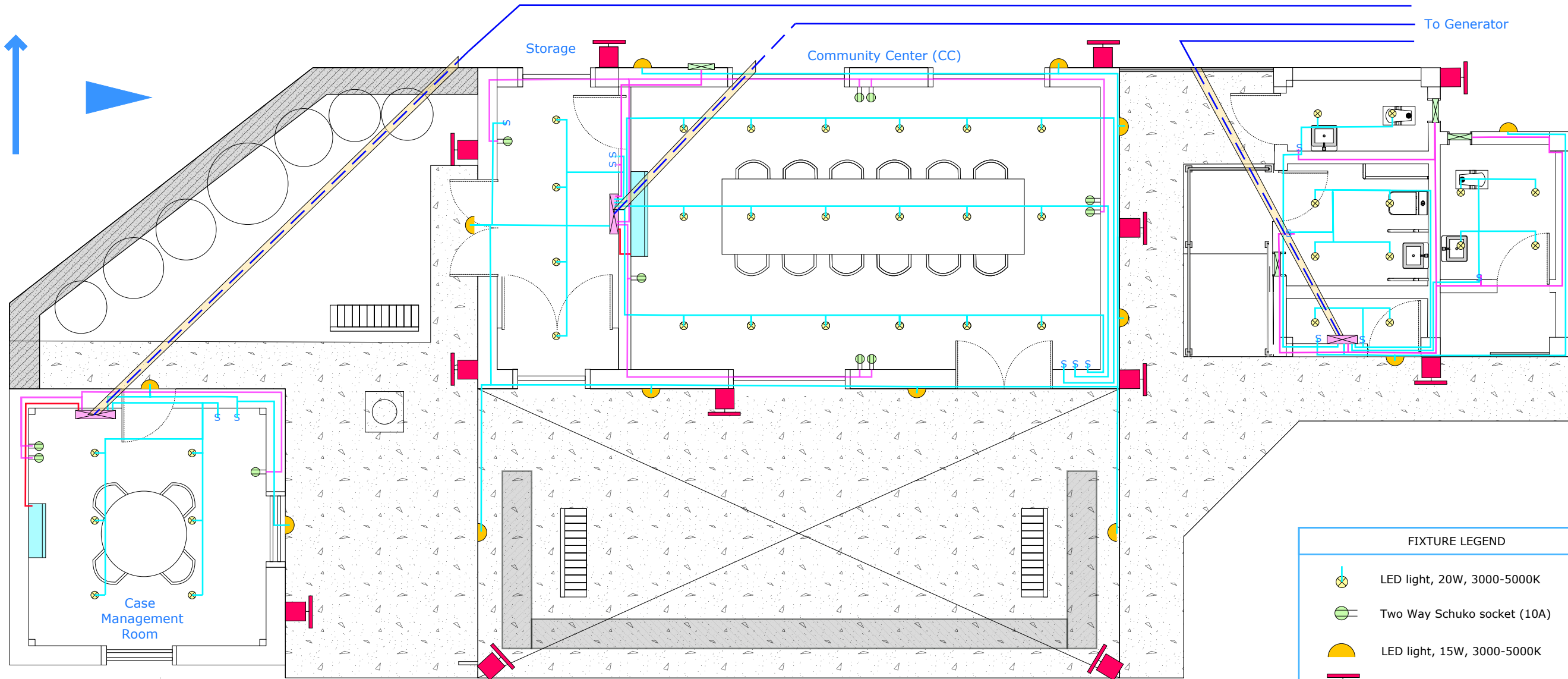
01 ELECTRICAL PLAN E SCALE: 1:70
